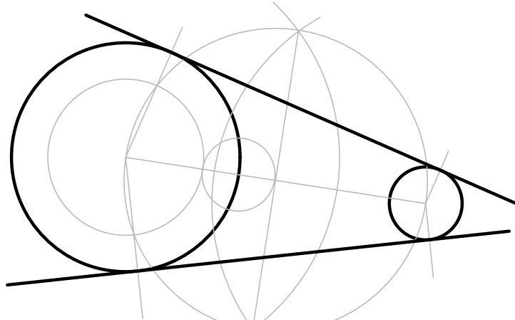
Tangentes exteriores a dos circunferencias
