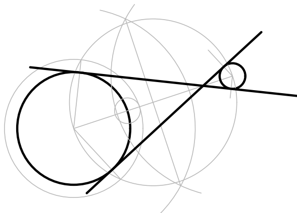
Tangentes interiores a dos circunferencias
