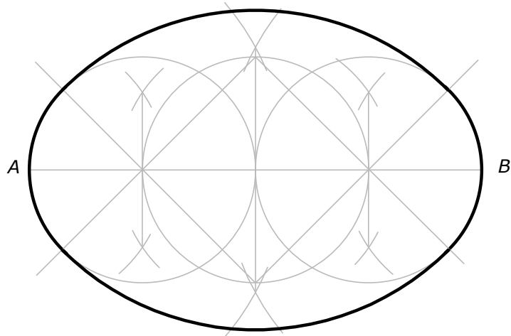
Óvalo dado el eje mayor AB
