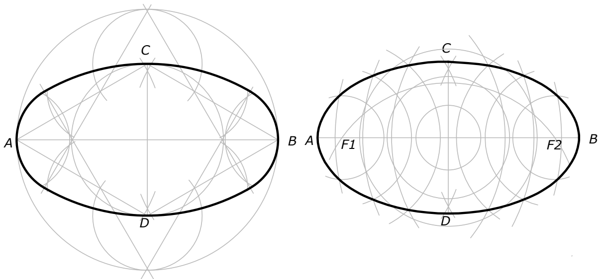
Óvalo y elipse dado eje mayor AB y menor AB
