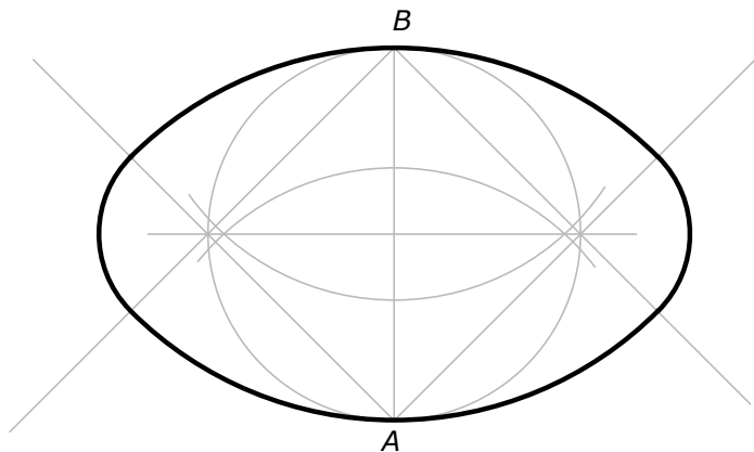
Óvalo dado eje menor AB
