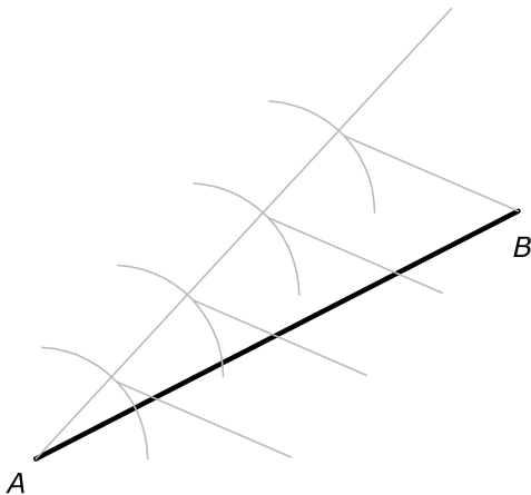
División AB en N partes
